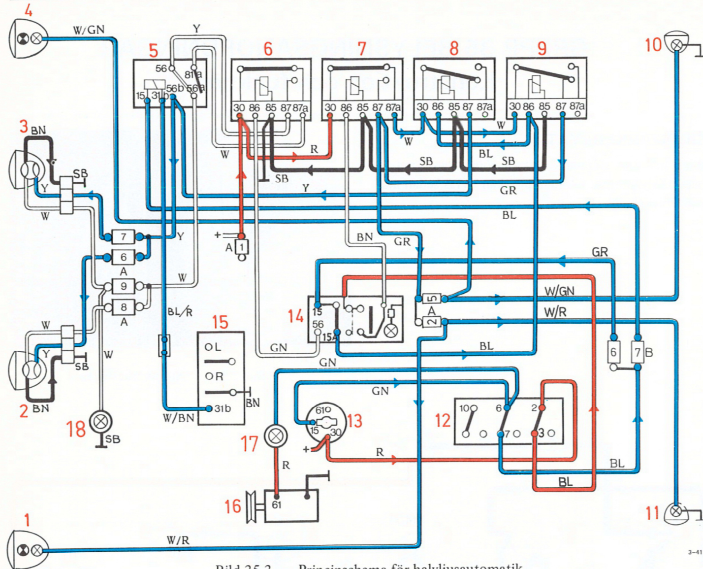
Bild 35-3. Principschema för halvljusautomatik
